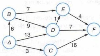
Рис. 3.7. Ориентированный граф
