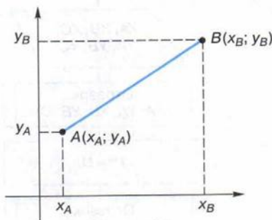
Рис. 2.11. Отрезок AB
