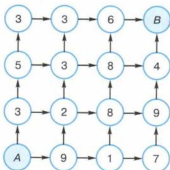
Рис. 3.17. Лабиринт
